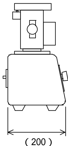
外観寸法図
